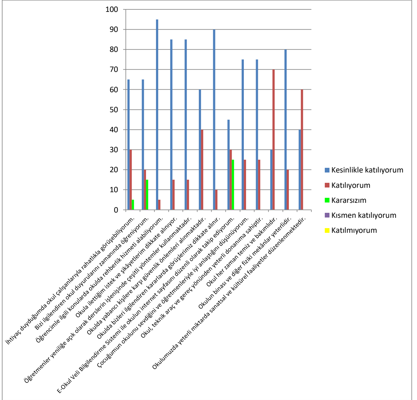
Şekil1. Veli Anketi
